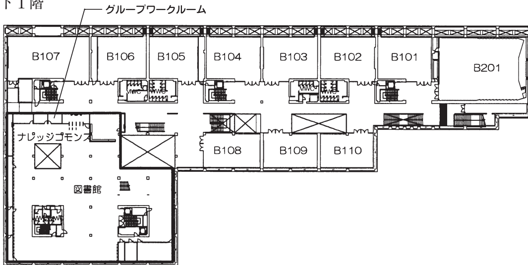
地下1階
